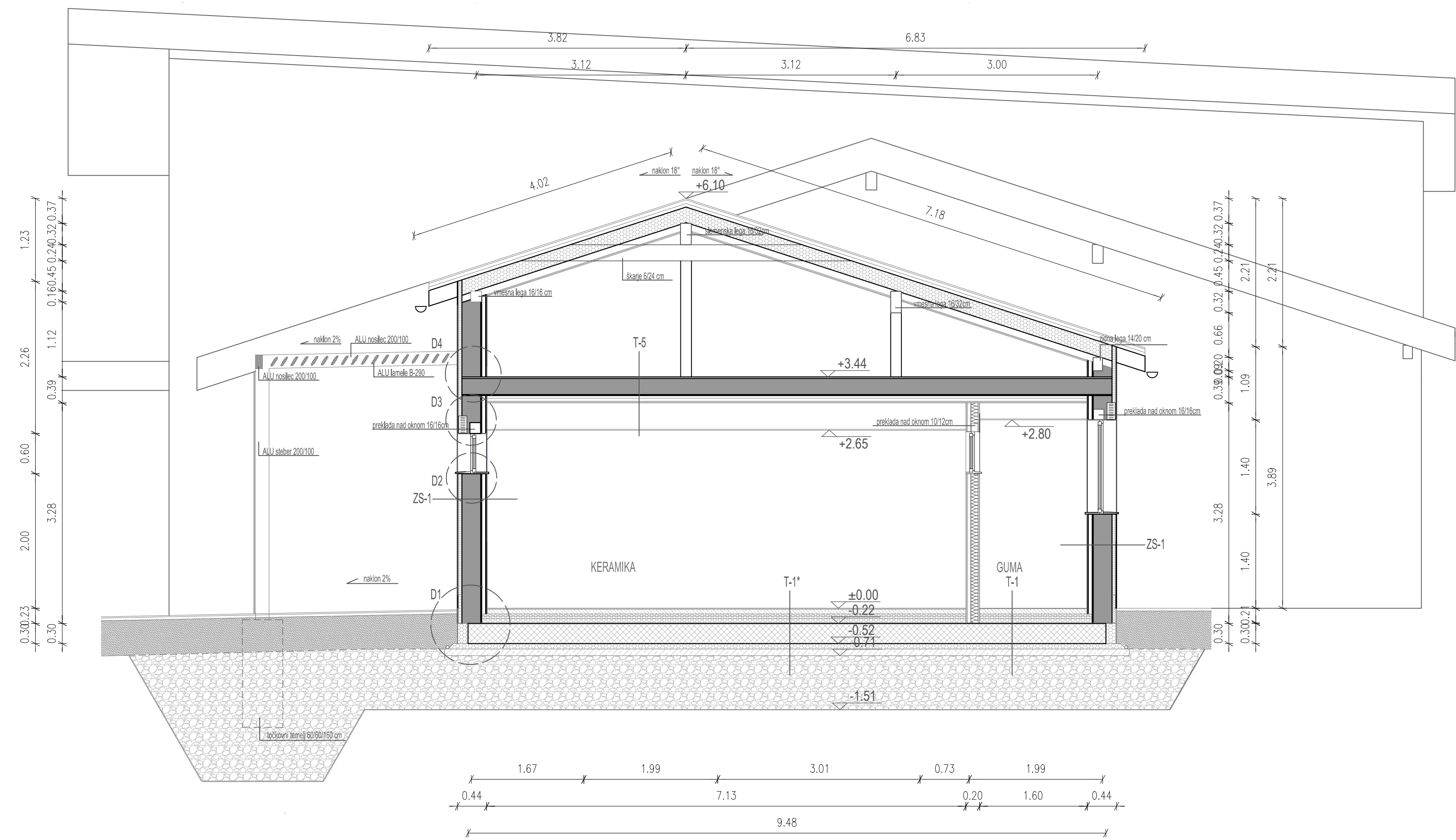
PREREZ A-A
